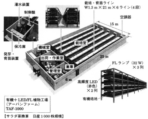
完全制御型植物工場概念図 (エスベックミック株式会社HPより改変)
